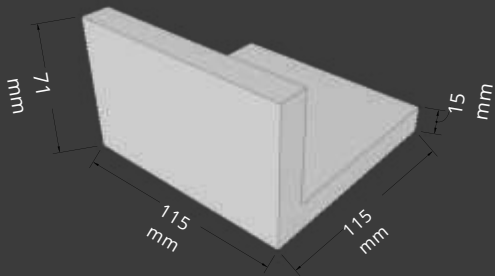
Kopfvollsteinwinkel 1 Header Edge Corner 1
