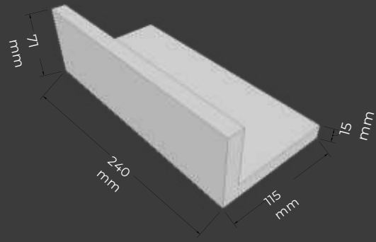
Läufervollsteinwinkel Edge Corner
