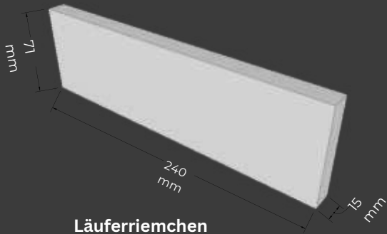
Läuferriemchen Thin Brick
