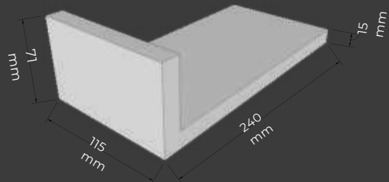
Kopfvollsteinwinkel 2 Header Edge Corner 2
